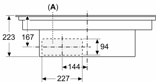
Mått i mm Frontvy
